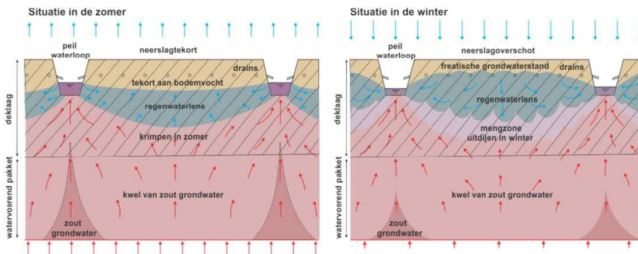
Figuur 3: Dynamiek grondwaterstroming in zomer- en winterperiode (Deltares, 2016).
