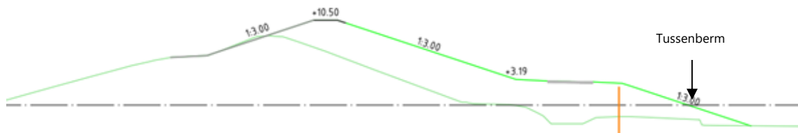
Afbeelding 2.21 Dwarsprofiel - Dorpsrand Zeedijk - Pluimpot-Mastgat (dp264 - dp268)
