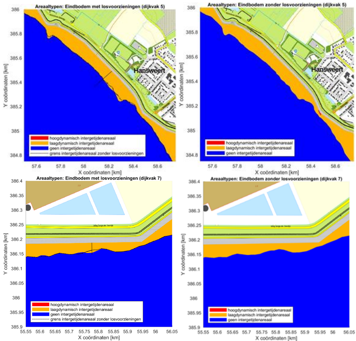
Afbeelding 5.5 Veranderingen in hoog- en laagdynamisch areaal met (links) en zonder (rechts) losvoorzieningen. Boven betreffen de modelresultaten voor dijkvak 5; onder voor dijkvak 7
